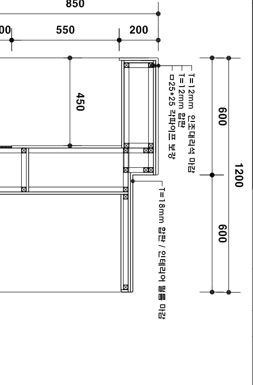
1 미디어라인 단면상세도 SCALE A1 1/20 A3 1/40
