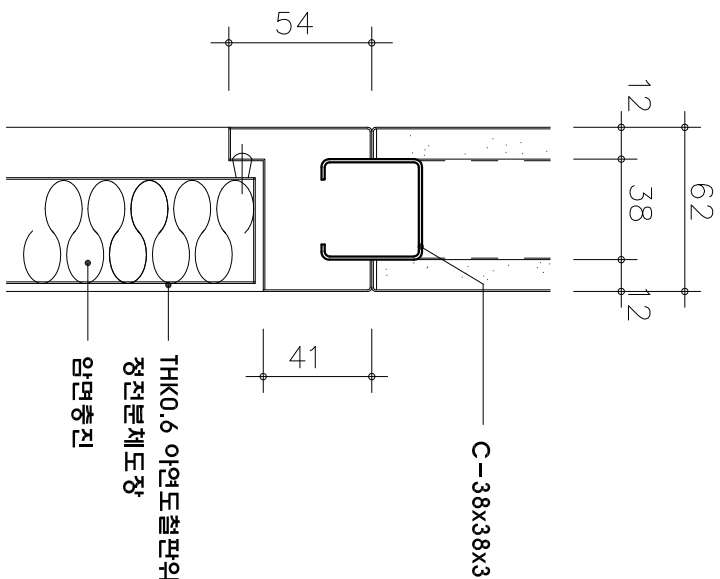
상세 "D" SCALE 1/3
