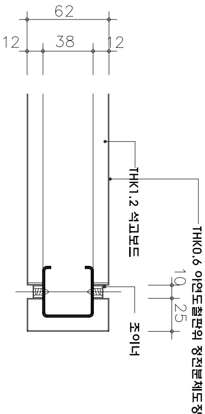
상세 "B" SCALE 1/3
