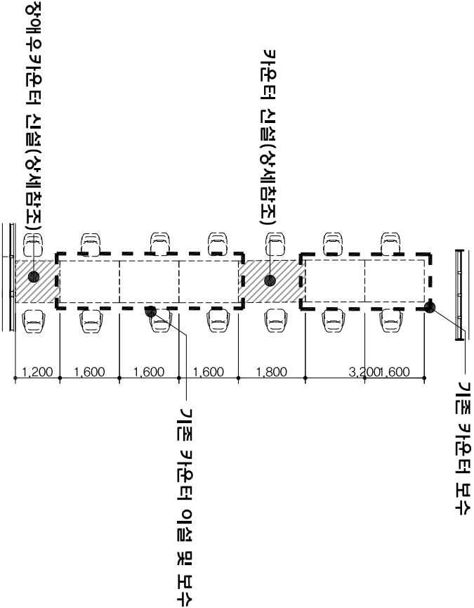
01 A 카운터 공사 범위도
