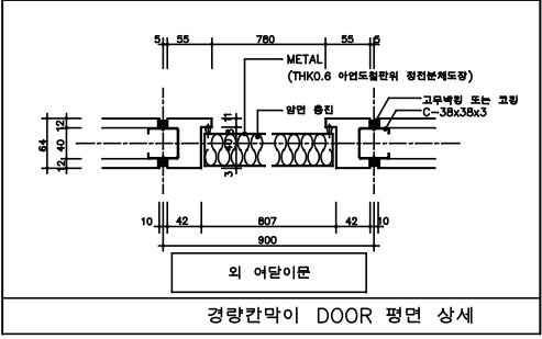
경량칸막이 DOOR 평면 상세
