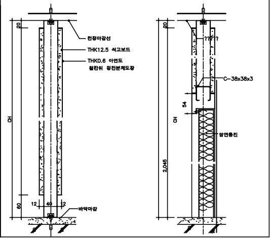
ATM 부스 상세
