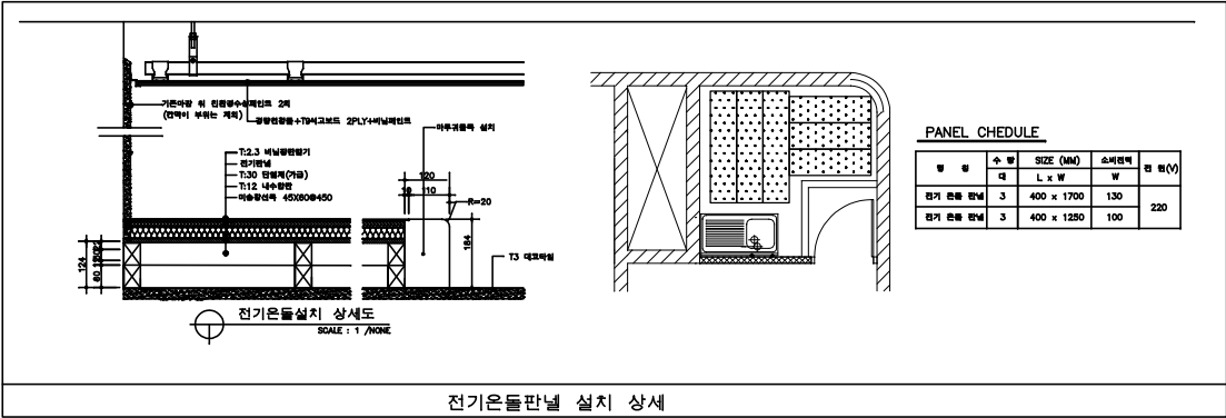
전기은들판넬 설치 상세
