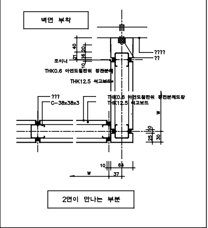
전기은들판넬 설치 상세
